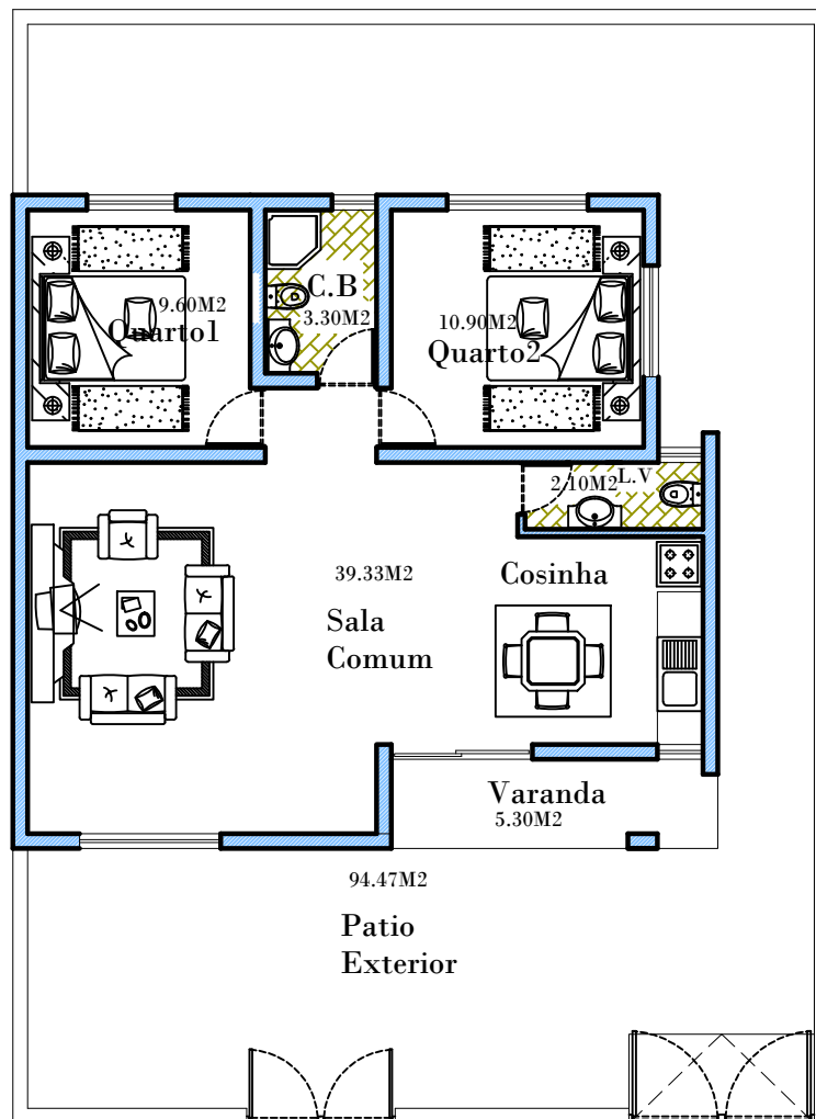
Planta do 1º Piso Moradia T2
